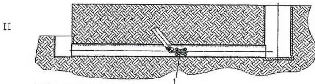
Auffräsen von Seitenkanalanschluss
