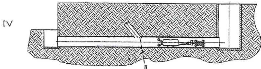
Sanierung des Seitenkanalanschlusses mittels Laminathut-Setzsystem (oder Verpresssystem)
