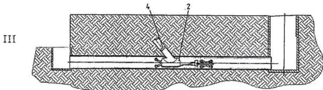
Sanierung des Seitenkanalanschlusses mittels Laminathut-Setzsystem (oder Verpresssystem)
